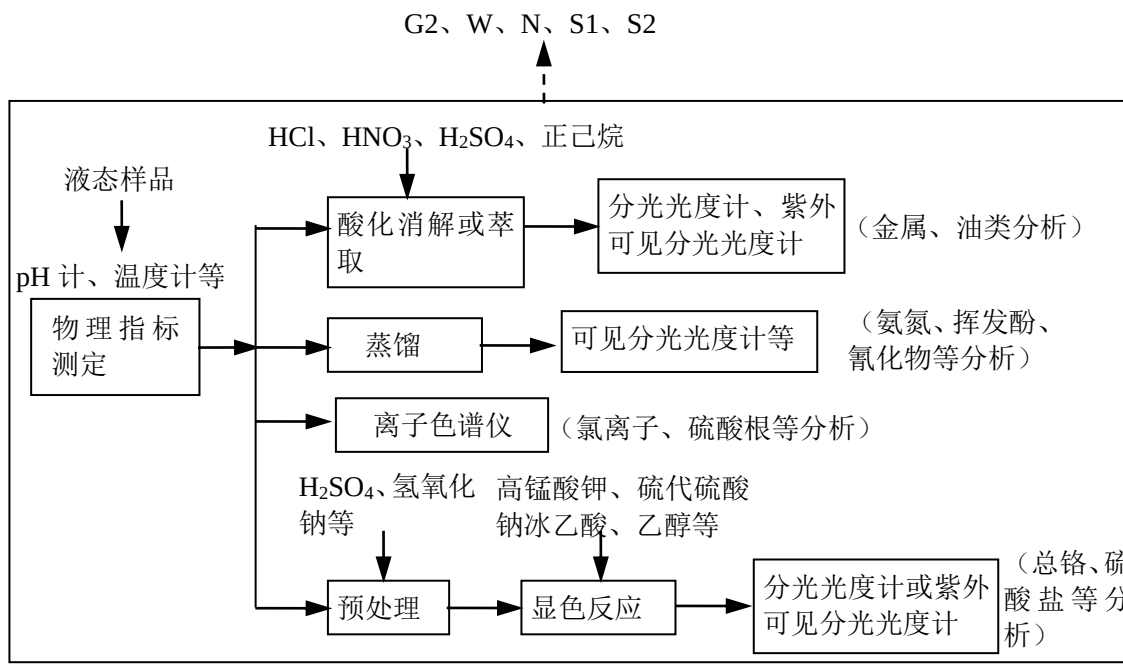
图 2-4 液态样品处理工艺流程
