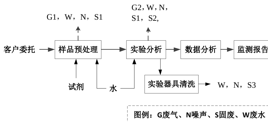
图 2-3 项目生产工艺流程及排污节点示意图
