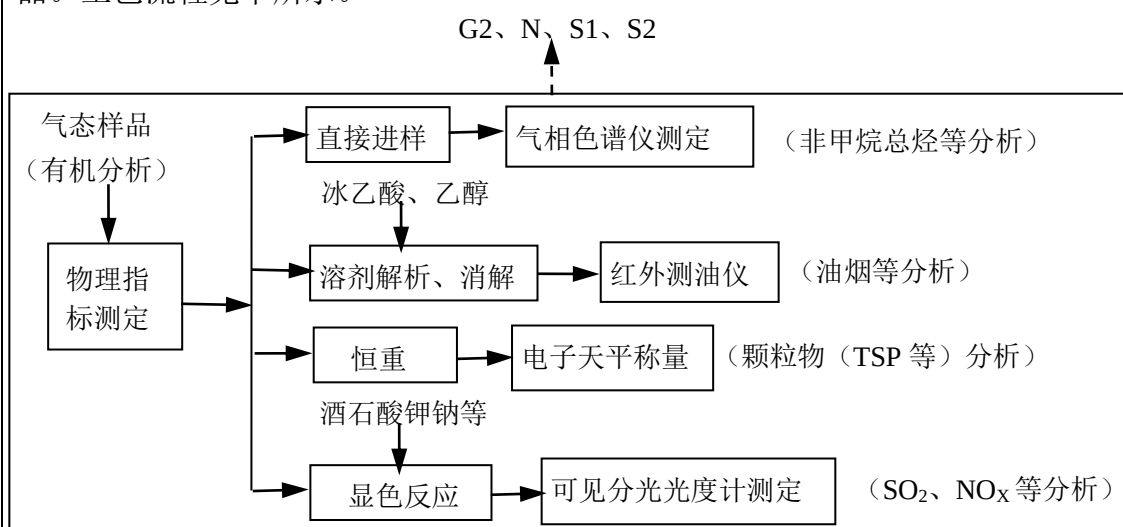
图 2-5 气态样品处理工艺流程
