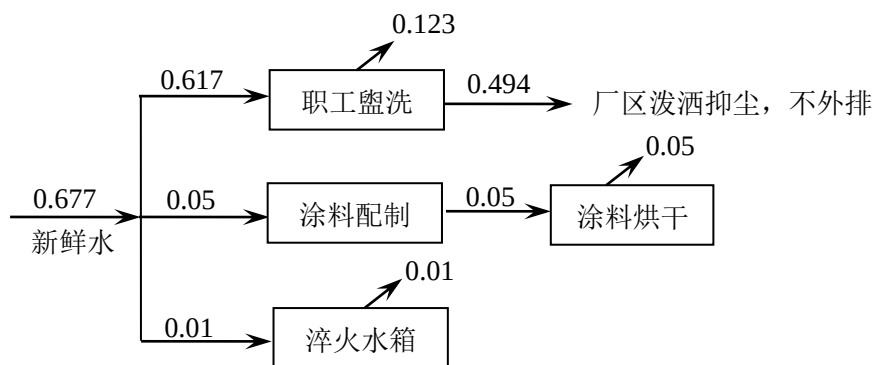
图 2-1 项目给排水平衡图 单位: \text{m}^3/\text{d}
