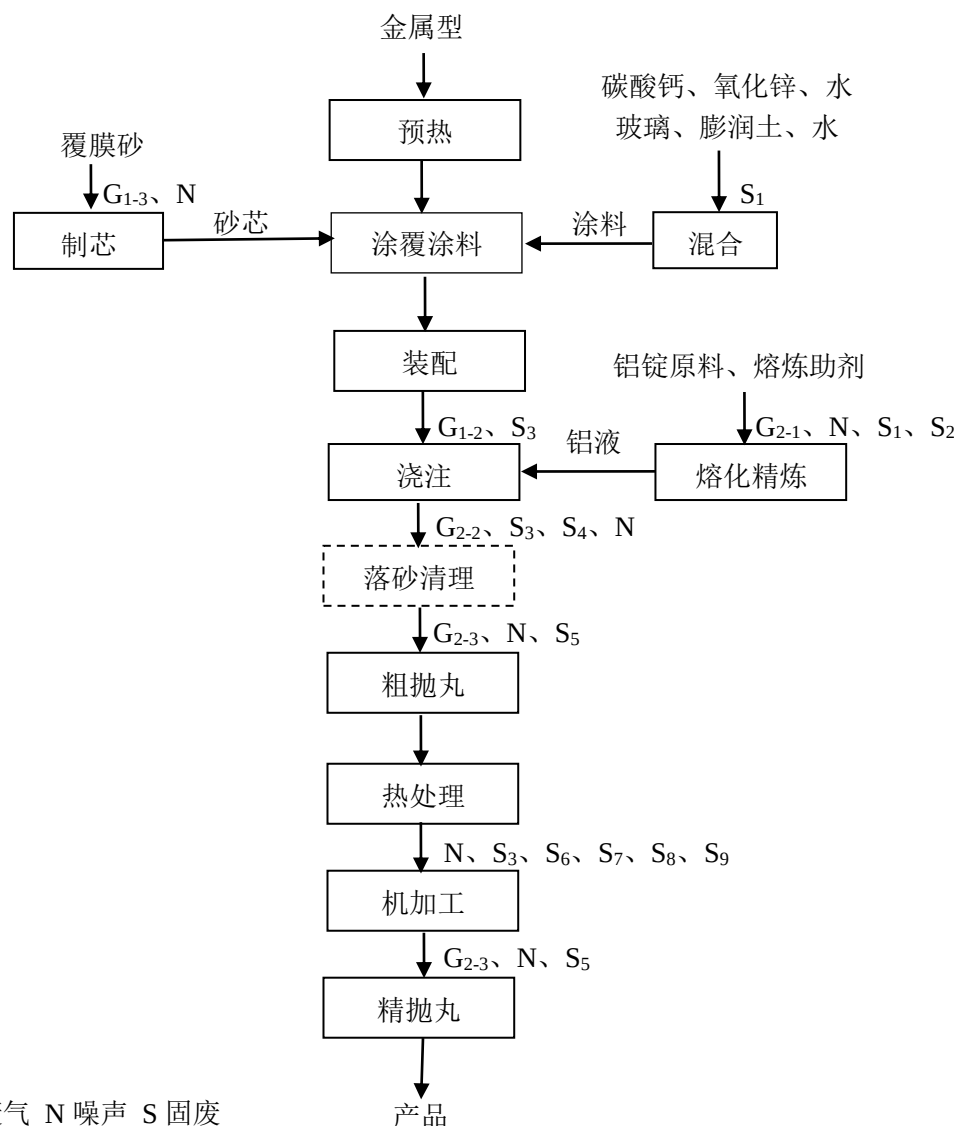
图 2-4 金属型铸造生产工艺流程及排污节点图
