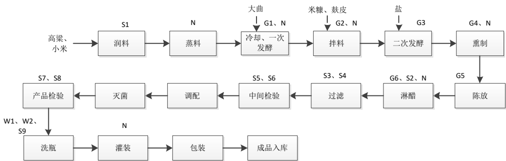
图 2-3 生产工艺流程图及排污节点
