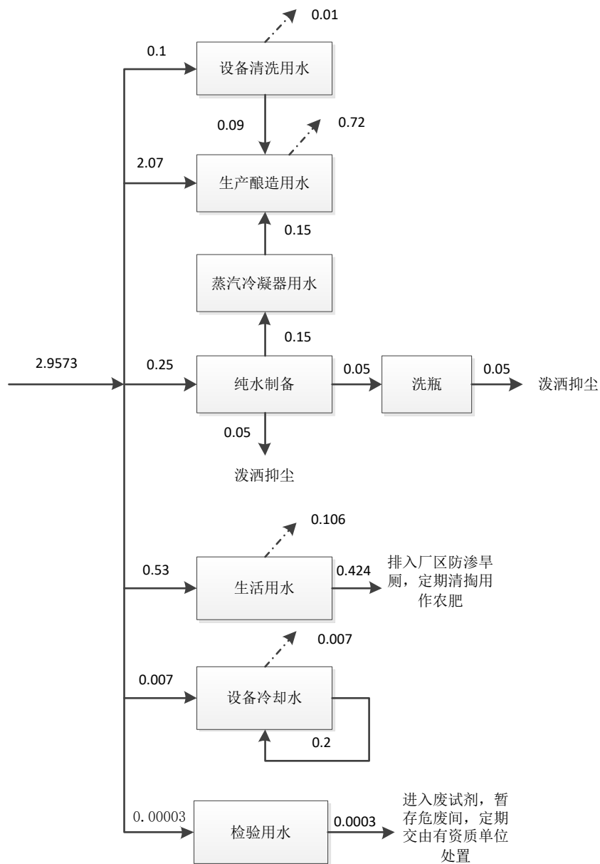
图 2-1 项目给排水平衡图 m³/d
