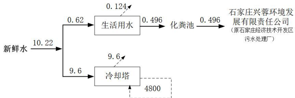
图 2-1 项目给排水平衡图 (单位 \text{m}^3/\text{d} )
